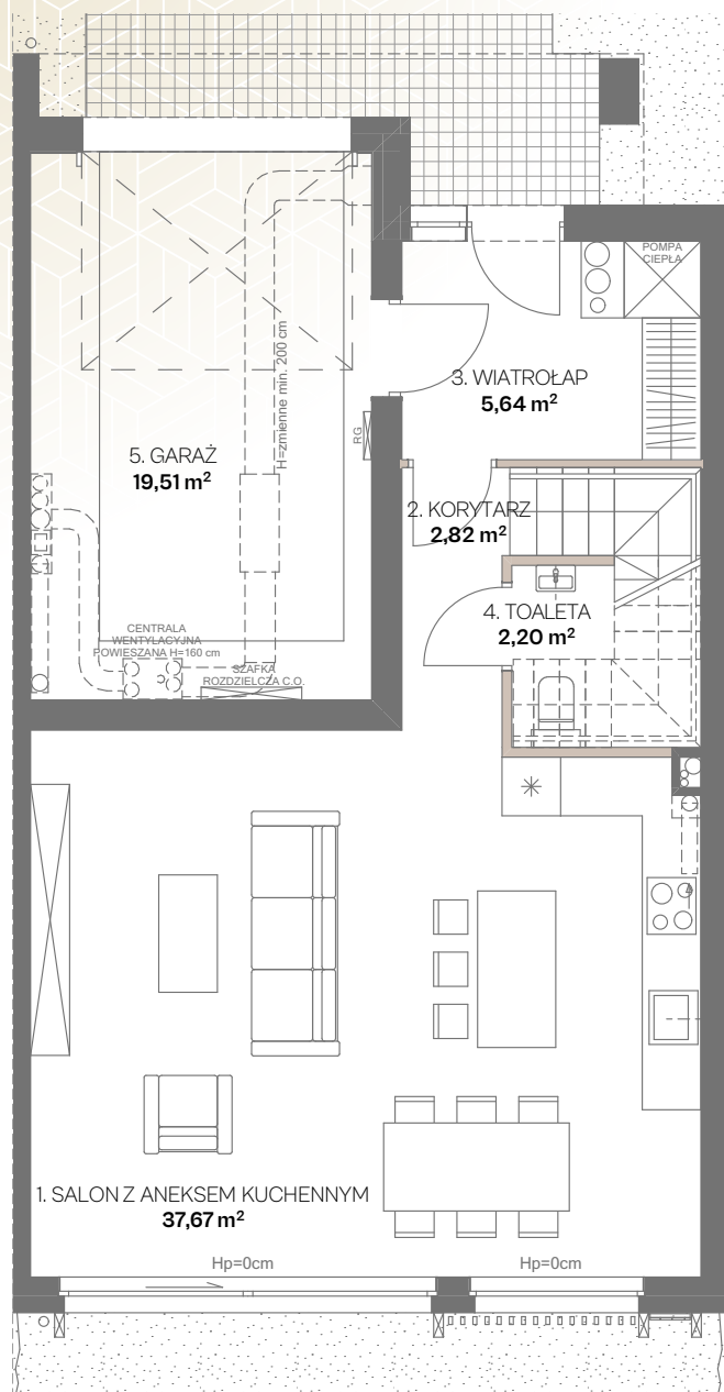
RZUT PARTERU
